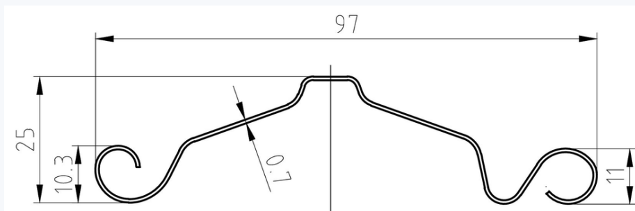
SECCIÓN TRANSVERSAL · COTAS EN MILÍMETROS (MM)
