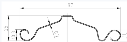
Mismo perfil europeo · cara perforada · cotas en mm
